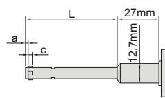
A型 6-12.5mm, 三点式 钢测量面
